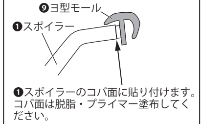
[ヨ型モール貼り付け断面図]
